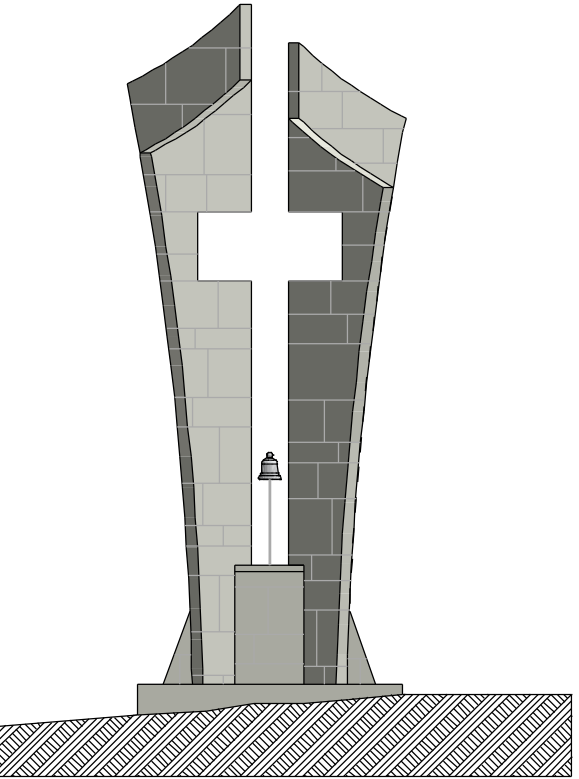
1:100 Ανατολικη Οψη
