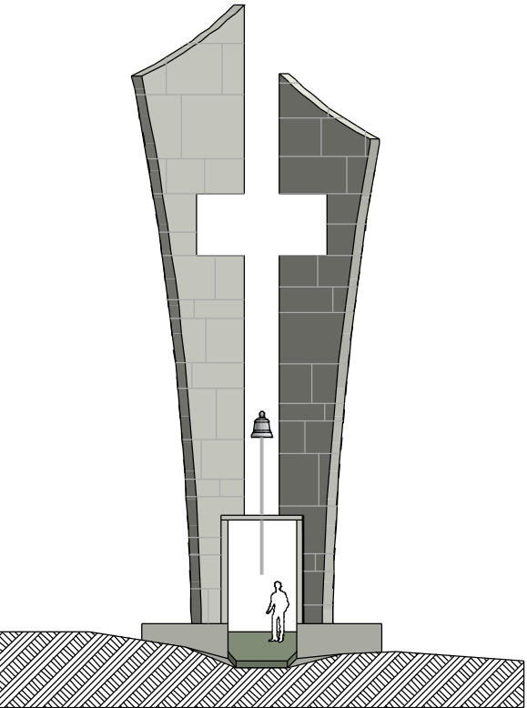
1:100 Νοτια Οψη
