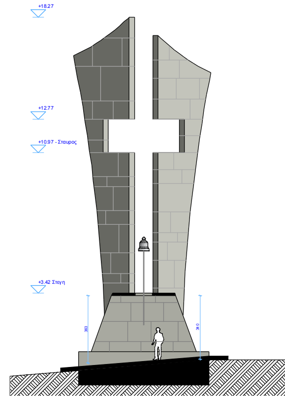
1:100 Τομη
