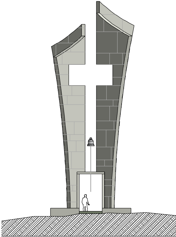
1:100 Βορεια Οψη
